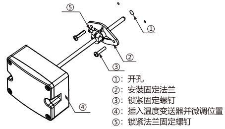
LFW10-2安装图
