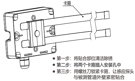
LFW10-5安装图
