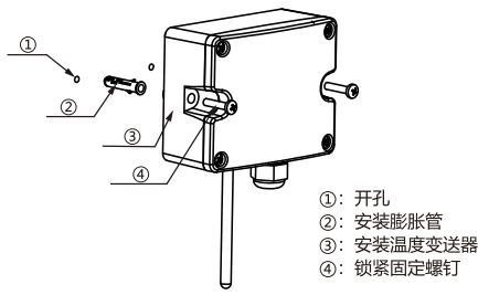
LFW10-1/4安装图
